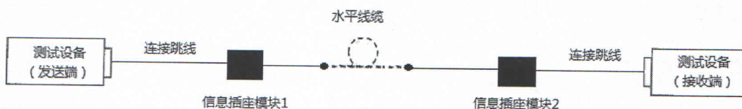
附图 1 测试连接示意框图
